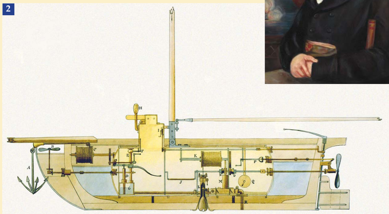
1. Портрет Роберта Фултона. Худ. Б. Уэст, 1809. 2. Чертеж подводной лодки Фултона «Наутилус».
