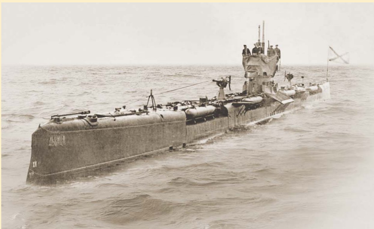
Подводная лодка «Львица» типа «Барс» в походе, 1915 г.
