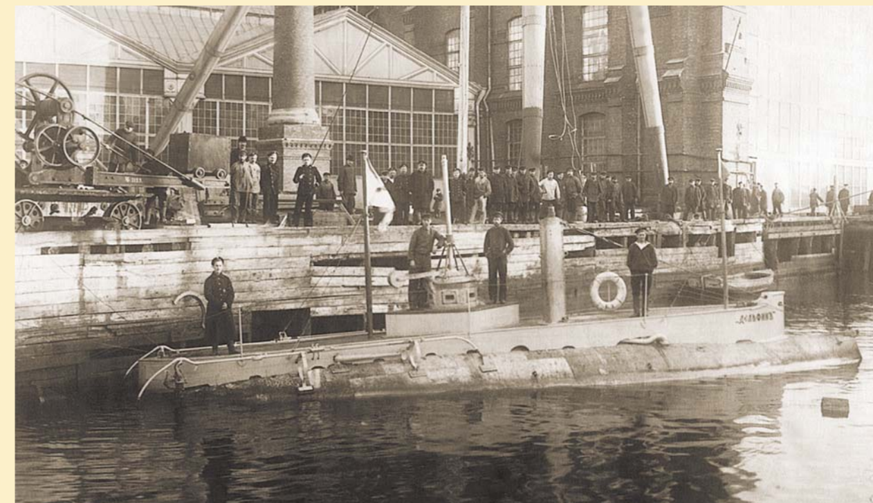
Подводная лодка «Дельфин» после модернизации у стенки Балтийского завода, 1904 г.
